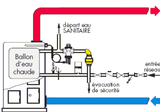
Installation de la soupape de sécurité thermique sur chaudière avec ballon incorporé
