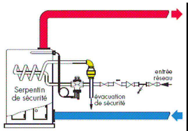
Installation de la soupape de sécurité thermique sur chaudière avec serpentin de sécurité
